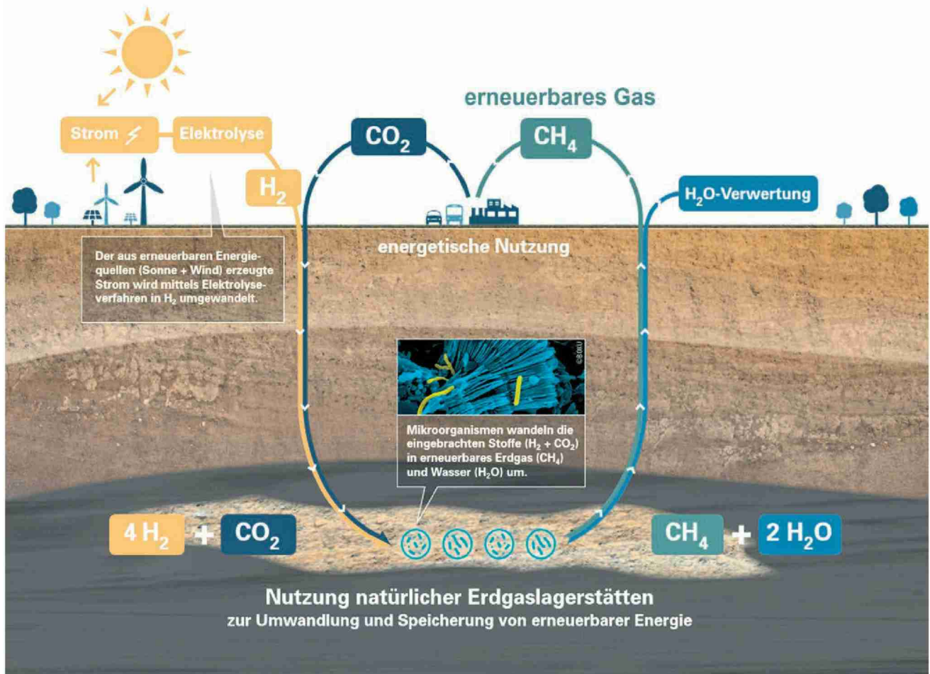
Schematische Darstellung einer Anlage, bei der erneuerbarer Wasserstoff (H 2 ) und Kohlendioxid (CO 2 ) in den durchlässigen Gesteinsschichten einer früheren Erdgaslagerstätte eingelagert und dort von Mikroorganismen in erneuerbares Gas umgewandelt werden.
